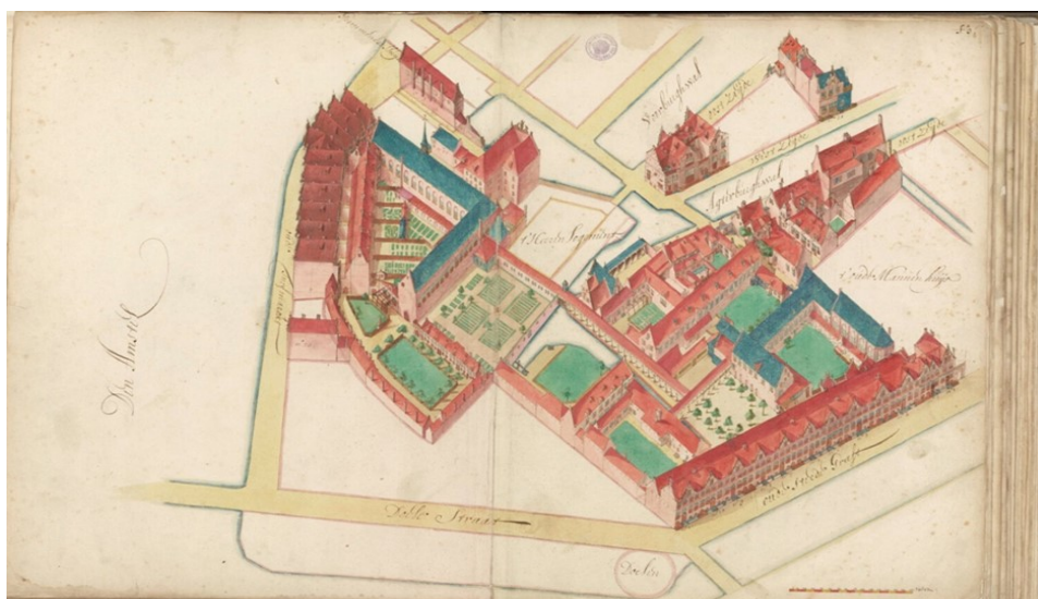
Afbeelding: Edifjci van de Gasthuysen (1628). Topografische tekening van het Sint-Pietersgasthuis waarop alle gebouwen in opstand getekend werden. Getekend door Balthasar Florisz van Berckenrode. Schaal ca 1:500.
